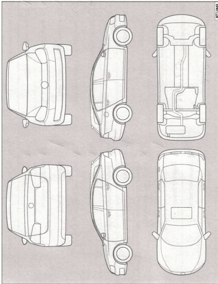
Obr. 7 Schematické zobrazení. Platí pro všechna vozidla a formy karoserie.
